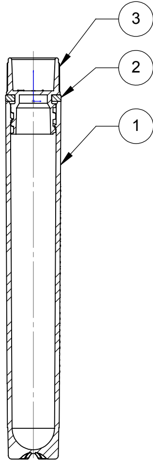
SECTION A-A
