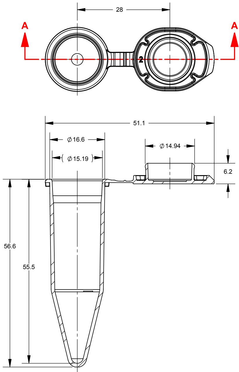
SECTION A-A SCALE: 1.5 : 1
