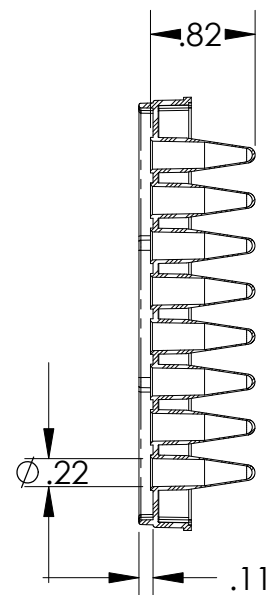
SECTION A-A
