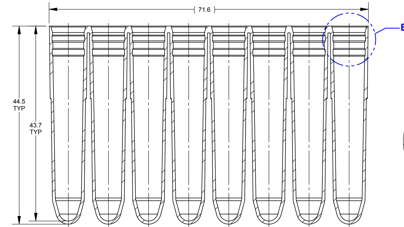
SECTION A-A SCALE: 2 : 1
