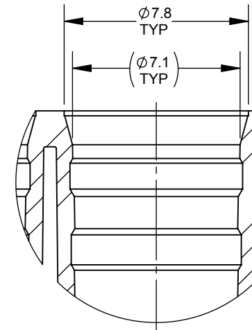
DETAIL B SCALE: 4.5 : 1
