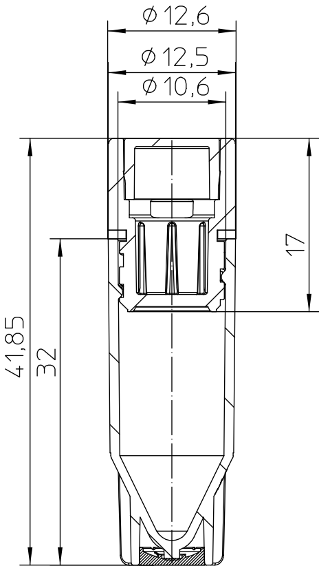
Schnitt A-A
